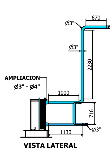
INTERCAMBIADOR PROPUESTO (Primera Etapa)
