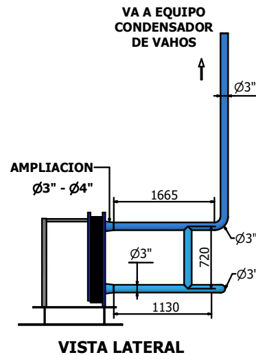
INTERCAMBIADOR EXISTENTE (Segunda Etapa)
