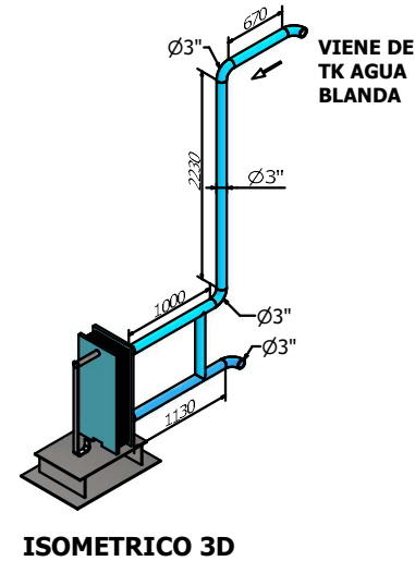
INTERCAMBIADOR PROPUESTO (Primera Etapa)
