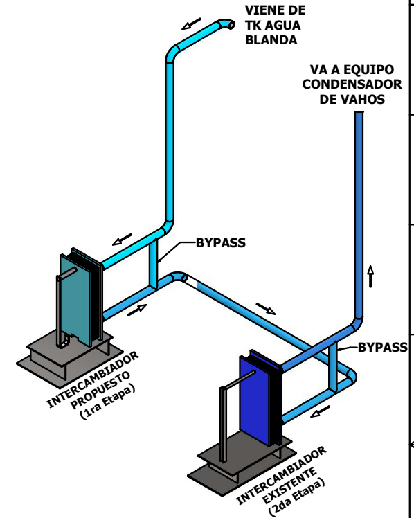
FLUJO DE AGUA BLANDA EN LOS INTERCAMBIADORES
