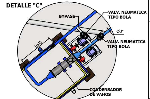
CONDENSADOR DE VAHOS (Tercera Etapa)
