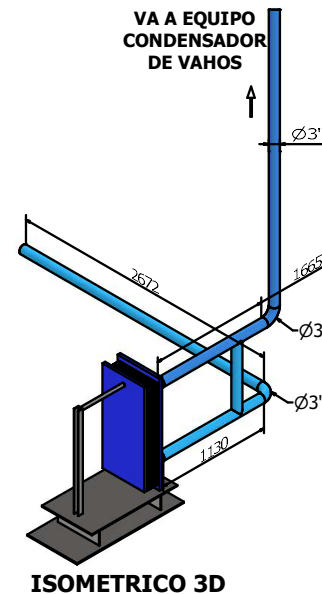
INTERCAMBIADOR EXISTENTE (Segunda Etapa)
